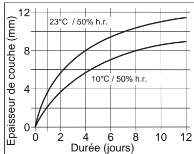
Diagramme 1: Vitesse de durcissement pour Sikaflex®-221
