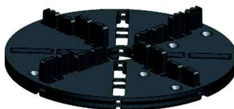
Gestapeltes VP-4 als 8mm Stelzlager
