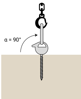
Abbildung 1 ausschließlich axiale Beanspruchung der Schraube bei einem Gehängewinkel von \alpha = 90^\circ .
