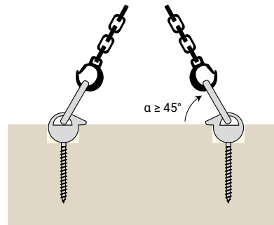
Abbildung 2 ausschließlich axiale Beanspruchung der Schraube durch passgenaue Topfbohrung bei einem Gehängewinkel von \alpha \geq 45^\circ .
