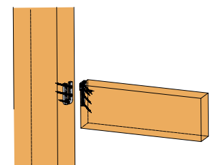
Stützenanschluss
